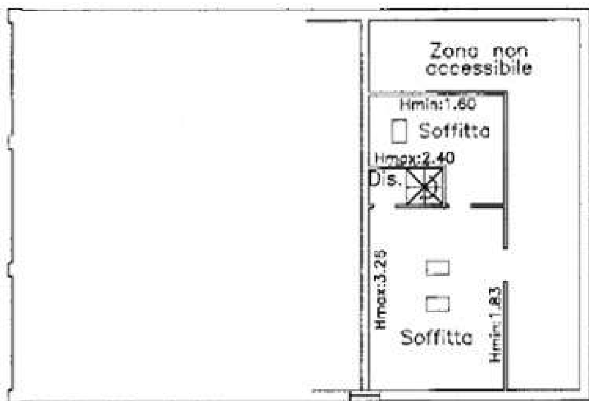
PIANTA PIANO SOTTOTETTO H_M = 2.54
