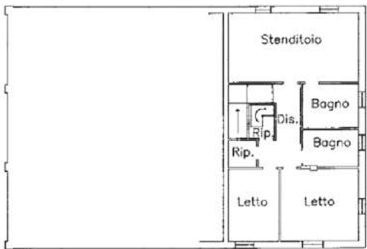
PIANTA PIANO PRIMO H= 2.80
