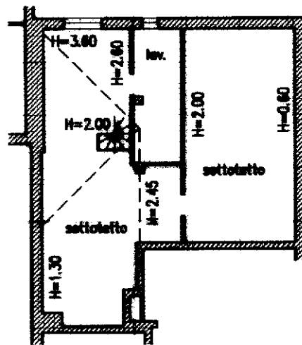
PIANTA TERZO PIANO
