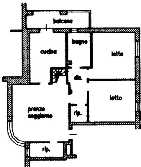
PIANTA SECONDO PIANO H=2.70
